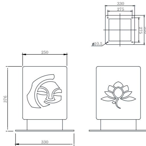
STS LED25W
